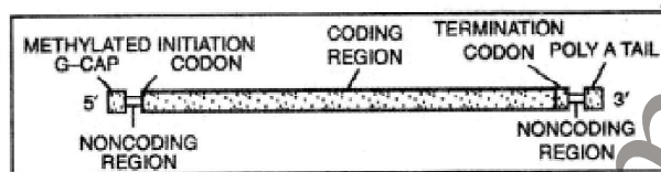
mRNA.
